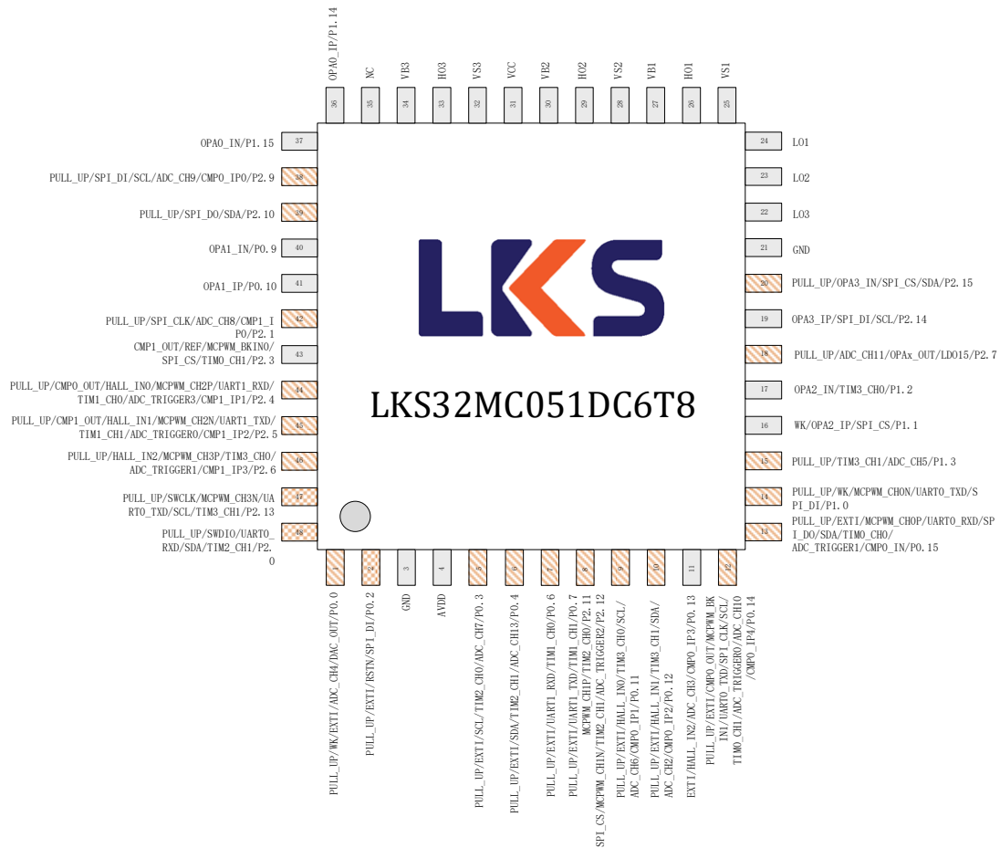
图 3-1 LKS32MC051DC6T8 管脚分布图
