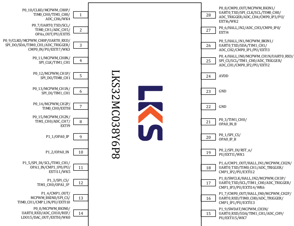
图 3-9 LKS32MC038Y6P8 管脚分布图
