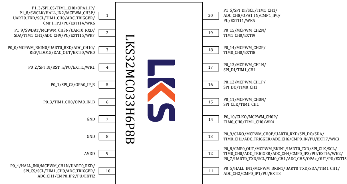
图 3-3 LKS32MC033H6P8B/LKS32MC033H6P8C 管脚分布图
