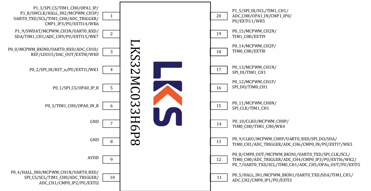
图 3-2 LKS32MC033H6P8 管脚分布图
