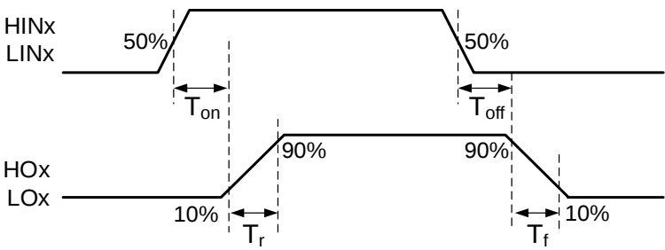
图 20-4 开关时序
